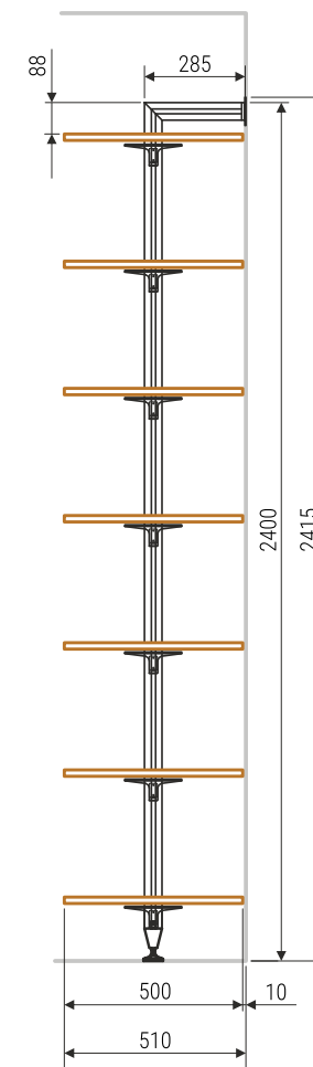
вид справа
