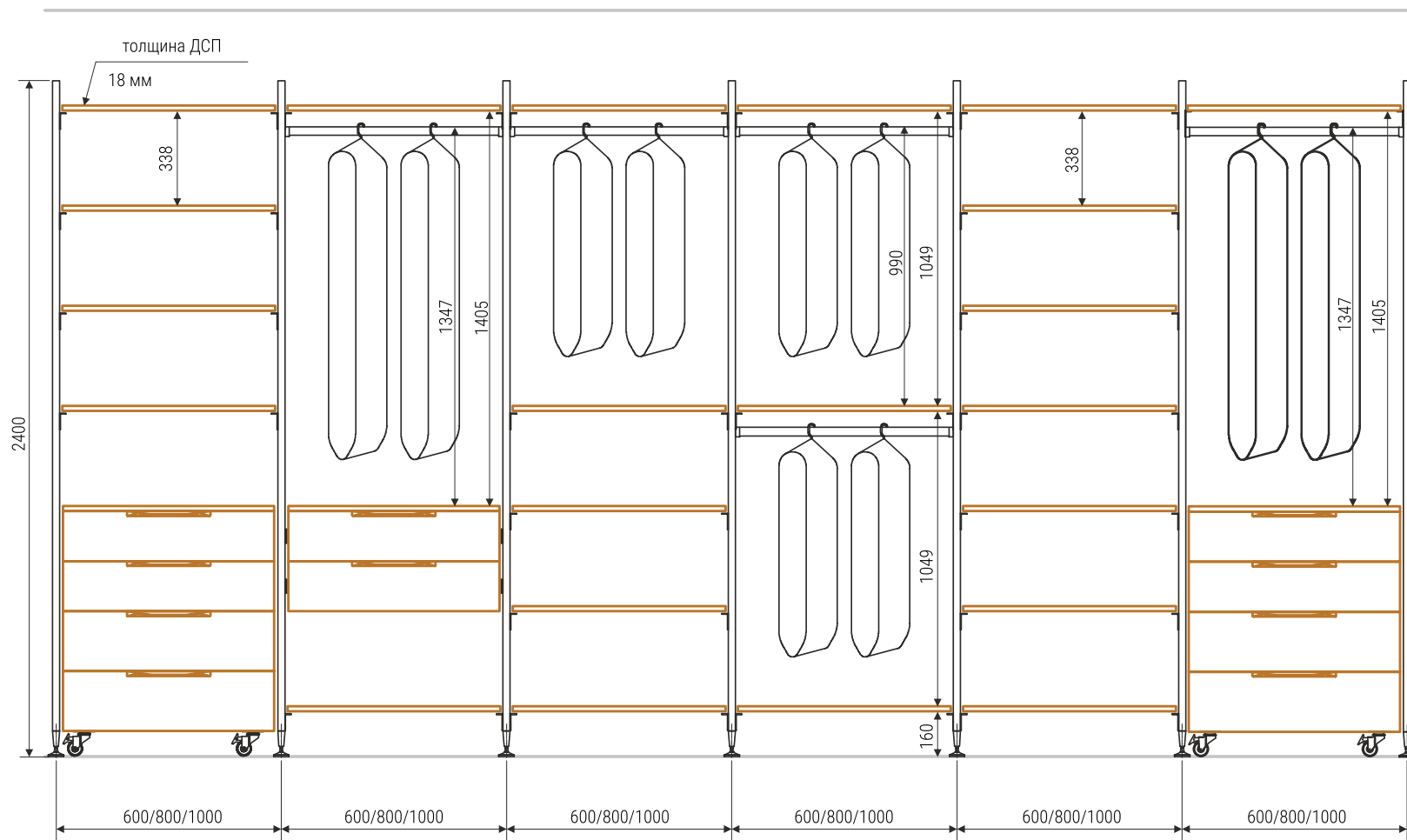
фронтальный вид
